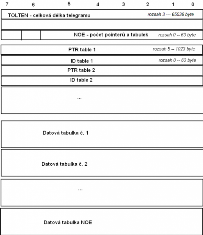
Obrázek 1 - Struktura telegramu
