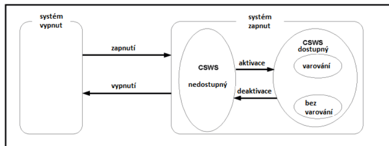
Obrázek 1 - Diagram přechodových stavů systému CSWS (obr. 1 normy)
