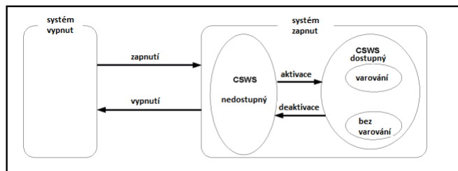
Obrázek 1 – Diagram přechodových stavů systému CSWS (obr. 1 normy)
