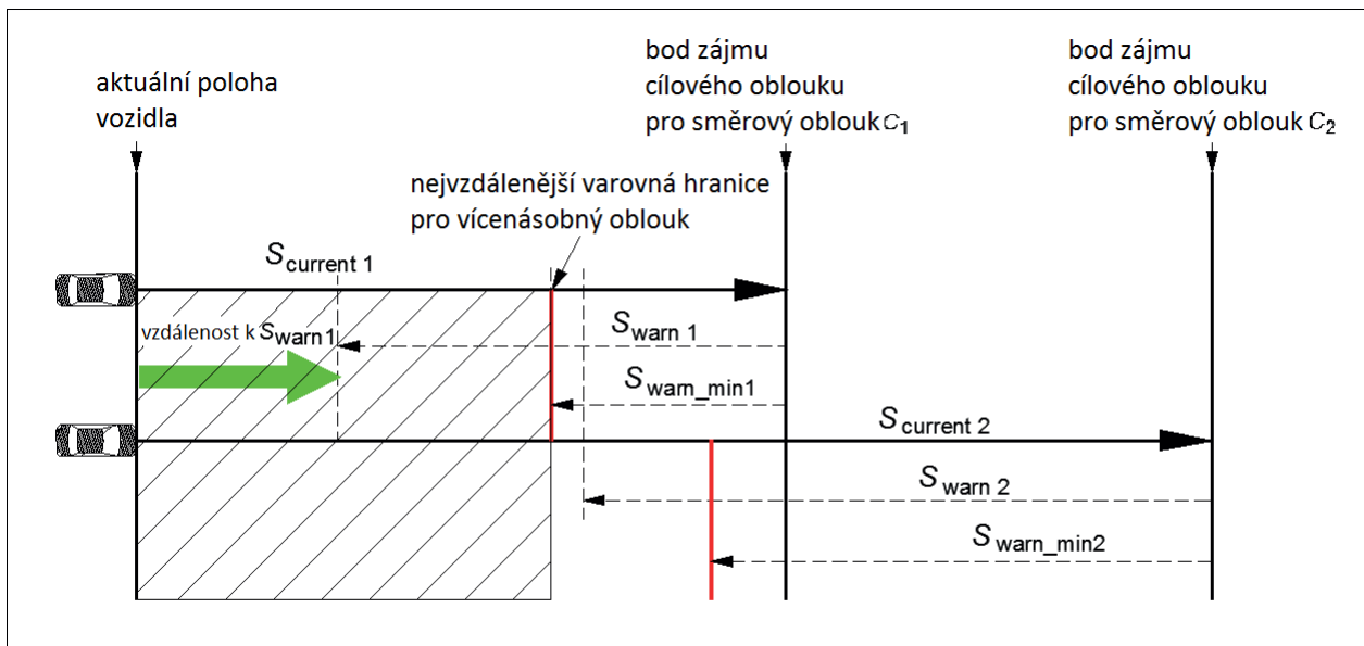
Obrázek 2 – Popis případu 1 (obr. 7 normy)
