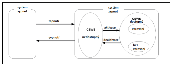
Obrázek 1 – Diagram přechodových stavů systému CSWS (obr. 1 normy)
