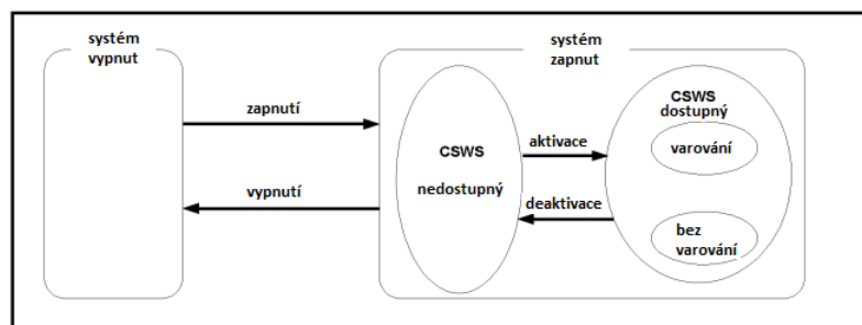
Obrázek 1 - Diagram přechodových stavů systému CSWS (obr. 1 normy)
