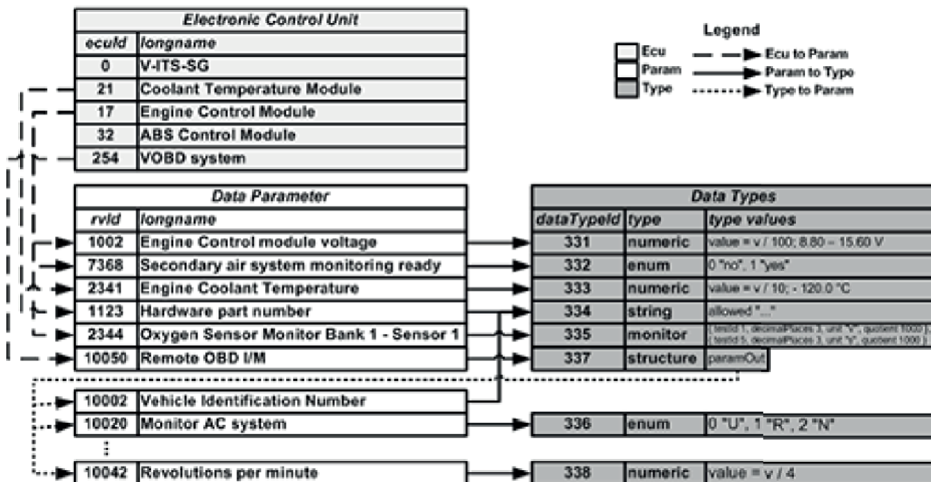
Obrázek 3 – Příklad VIDF (obr. A.1 normy)
