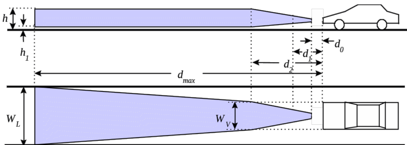
Obrázek 3 – Oblast detekce
