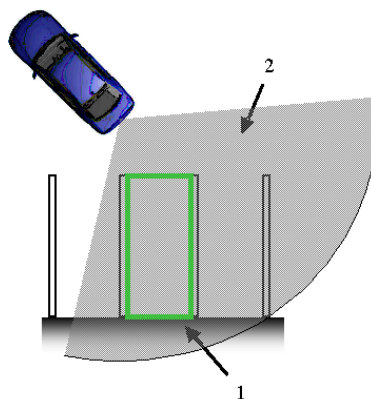
Obrázek 5 – Rozpoznání volného cílového parkovacího místa pro kolmé parkování (obr. C.2 normy)
