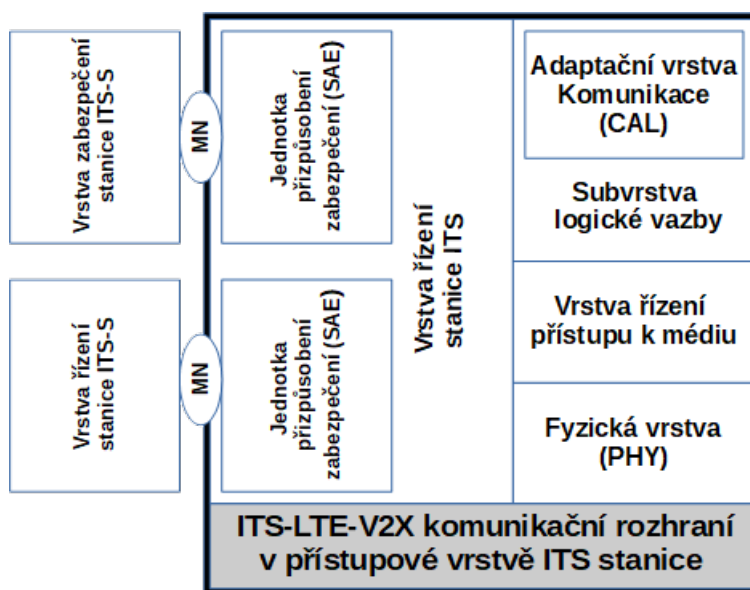
Obrázek 2 - Architektura komunikačního rozhraní LTE-V2X (obr. 2 normy)
