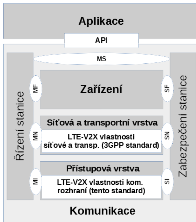
Obrázek 3 - LTE-V2X funkcionalita v rámci stanice ITS (obr. 3 normy)
