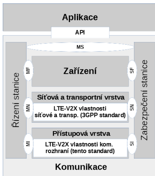
Obrázek 3 - LTE-V2X funkcionalita v rámci stanice ITS (obr. 3 normy)
