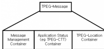
Obrázek 1 TPEG CTT struktura
