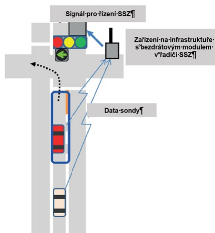
Obrázek 3: Schéma řízení pro levé odbočení (Obr. 3 normy)
