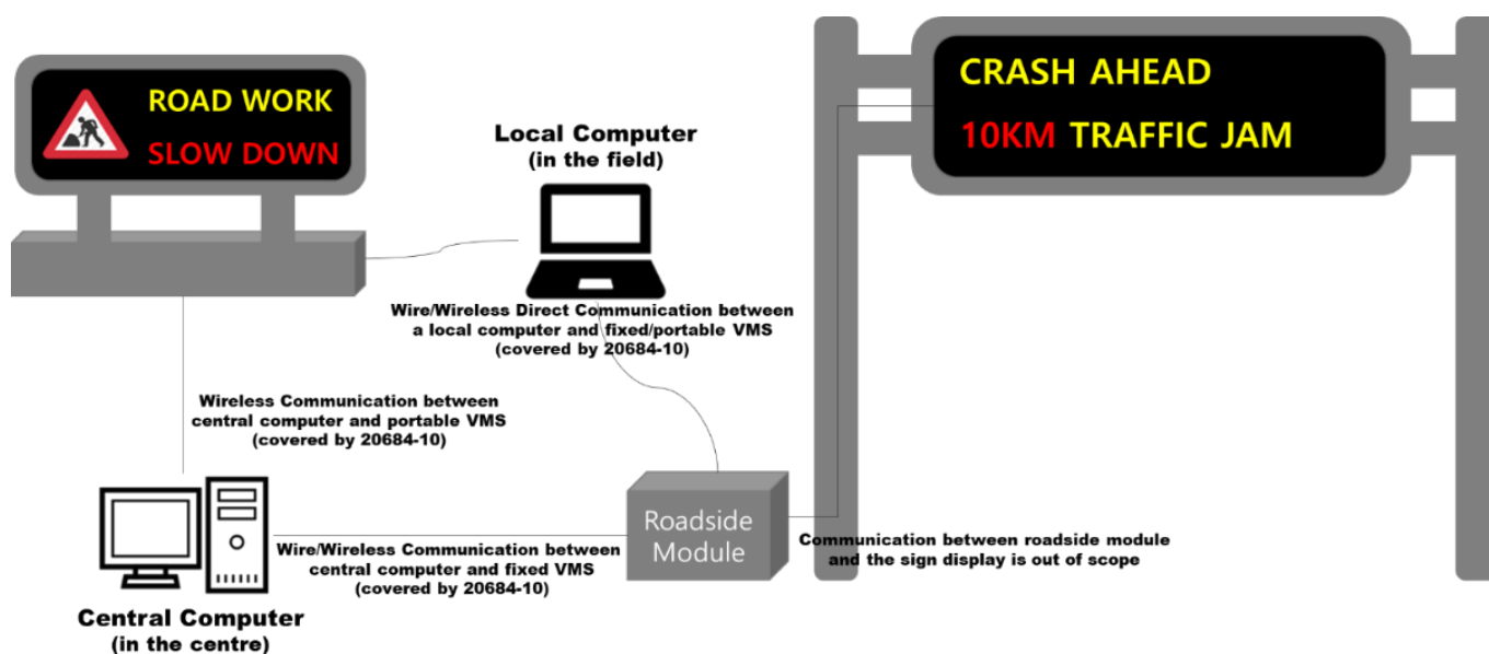
Obrázek č. 1 - Fyzická architektura (Obrázek č.1 popisovaného dokumentu)
