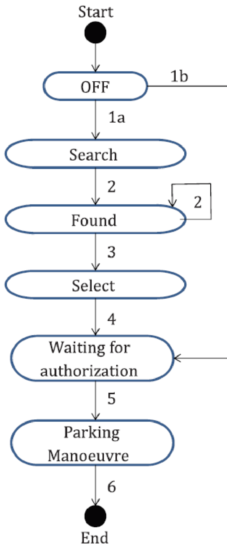
Obrázek 3 - Diagram provozních stavů PAPS při parkování (obr. 7 normy)
