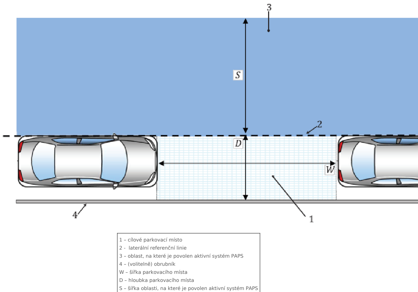
Obrázek 1 - Geometrie podélného parkovacího místa (obr. 1 normy)
