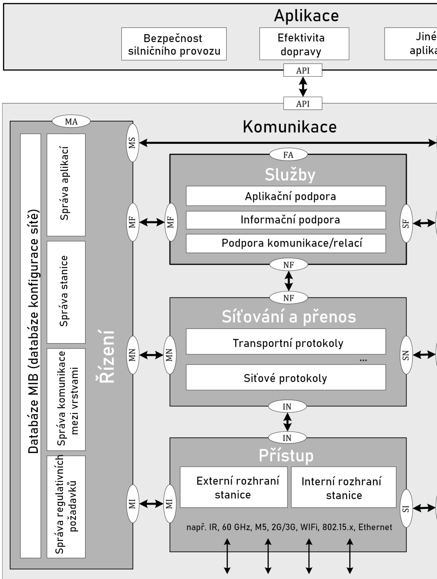
Obrázek 3 – Architektura pro komunikační profil a výběr cesty (obrázek 12 normy)
