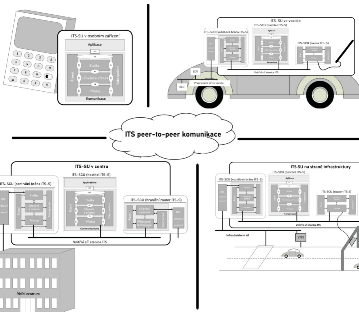
Obrázek 4 - Typická realizace jednotek ITS-SU (obrázek 29 normy)
