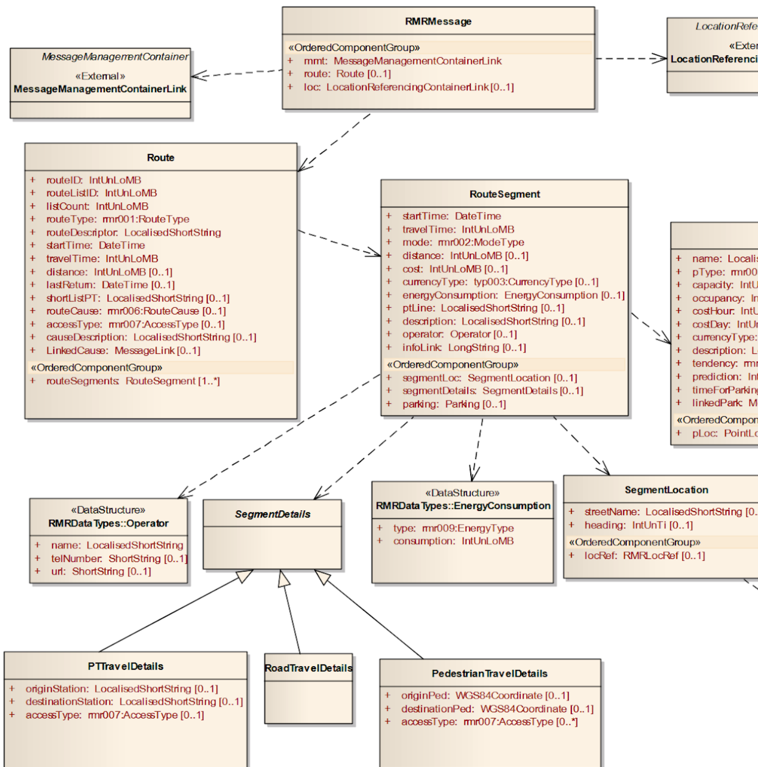
Obrázek 1 - UML model tříd aplikace RMR (obrázek 2 normy)
