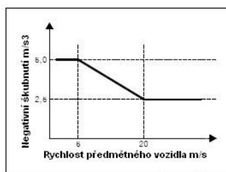
Obrázek 6 - Maximální zpomalení
