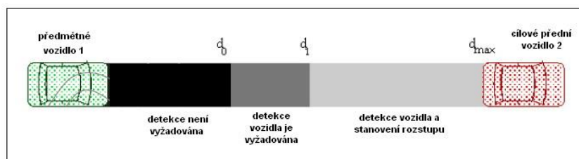
Obrázek 3 - Detekční zóny
