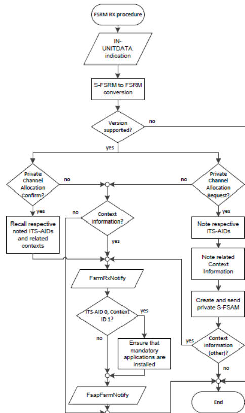
Obrázek 3 - příklad algoritmu zpracování FRSM (obr. 8 normy)
