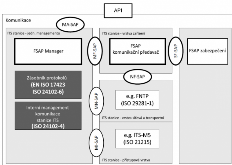
Obrázek 1 - Referenční architektura FSAP (obr. 4 normy)
