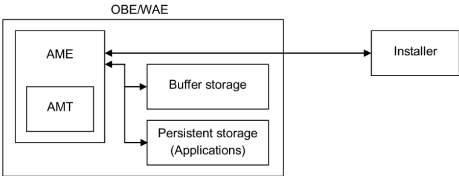
Obrázek 2 - Jednotky aplikačního managementu OBE/WAE
