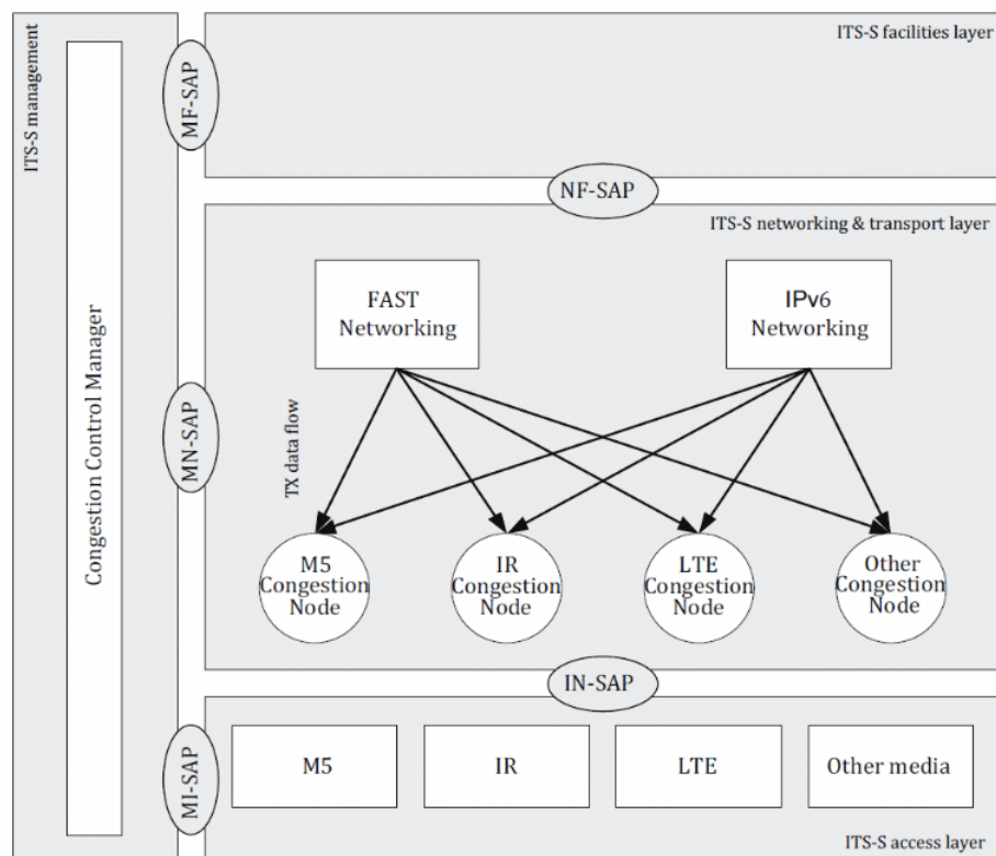
Obrázek 1 – architektura řízení datových front
