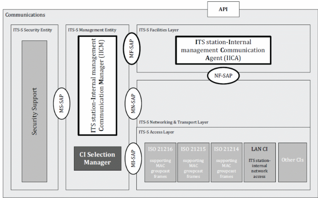
Obrázek 2 – referenční architektura
