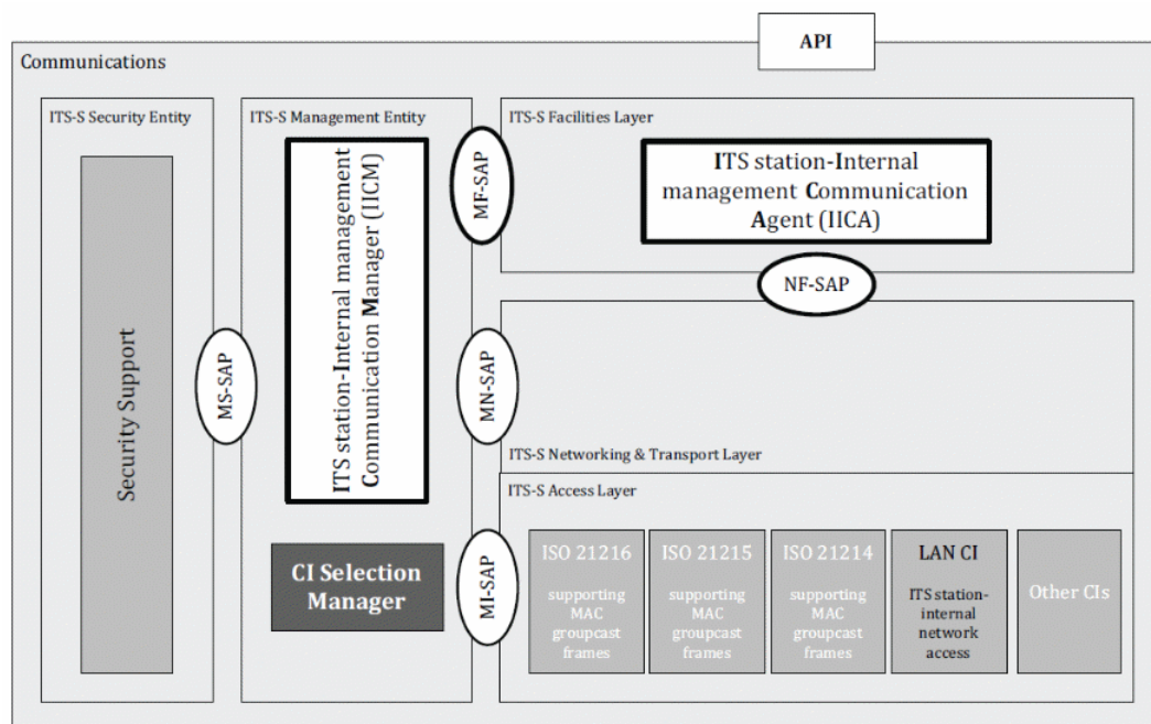
Obrázek 2 - referenční architektura
