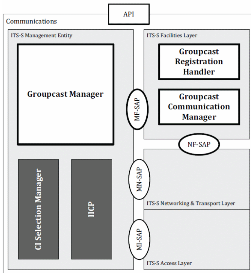
Obrázek 4 – referenční architektura
