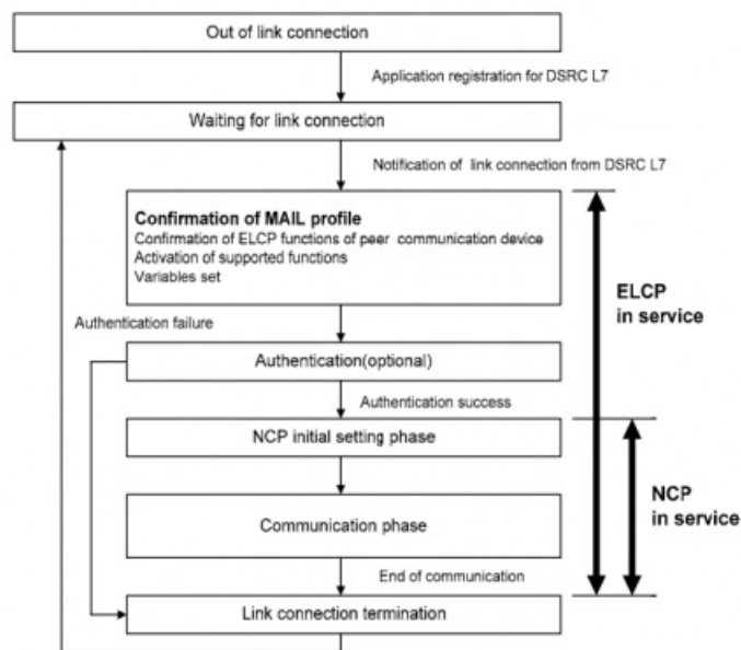
Obrázek 3 – Procedura MAIL
