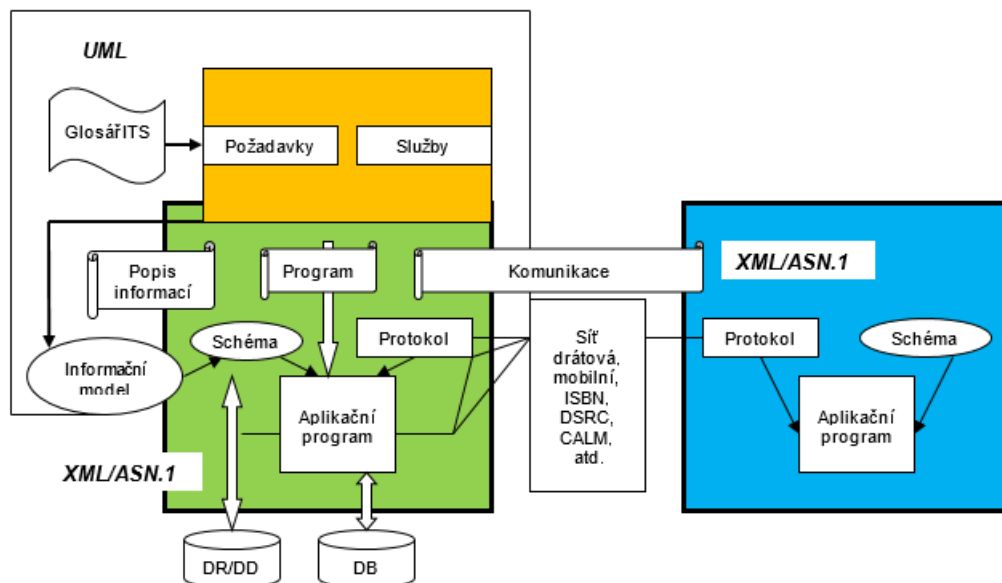
Obrazek 1 – Funkcionalita XML v systémech ITS
