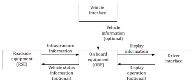
Obrázek 1: Uspořádání systému
