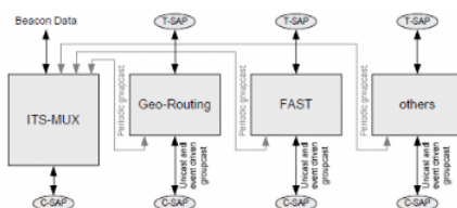
Obrázek 13 – Architektura protokolu ITS-MUX
