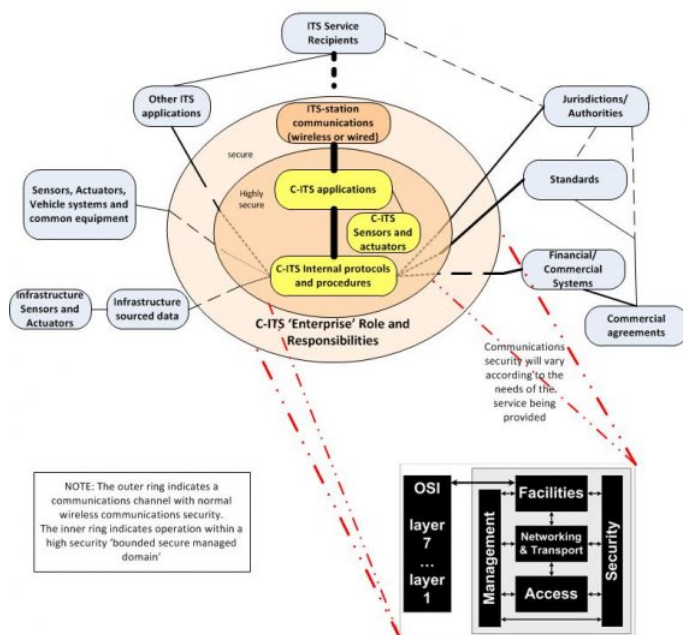
Obrázek 1: Schéma hranic základního systému (ISO 17427-1) (obr. 1 normy)
