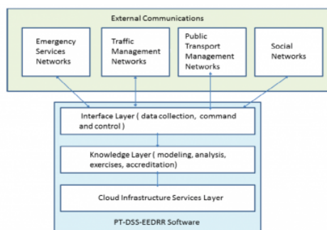
Obrázek 5 - Centralizovaná architektura PT-DSS EEDRR (obr. 3 normy)
