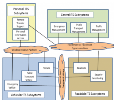
Obrázek 4 - Subsystém ITS v interakci s PT-DSS EEDRR (obr. 2 normy)
