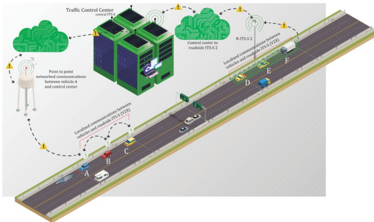
Obr. 1 (obrázek 2 normy): Upozornění využívající hybridní komunikaci
