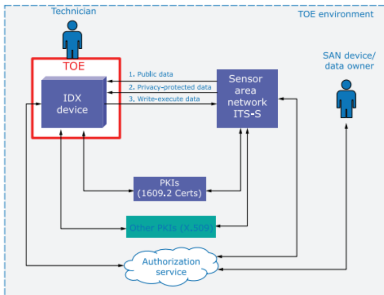
Obrázek 1 (obrázek 8 normy): Systémový pohled na "cíl vyhodnocení"
