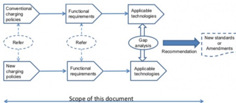
Obrázek 1 – Předmět tohoto dokumentu (obrázek 1 normy)
