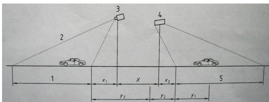
Obrázek 4 – Umísťování proměnných dopravních značek s ohledem na pozice kamer
