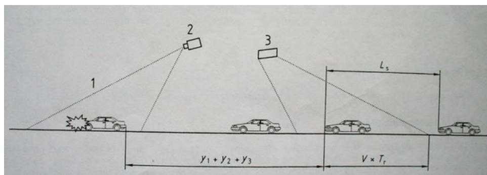
Obrázek 5 – Reakční čas systému s ohledem na vzdálenost
