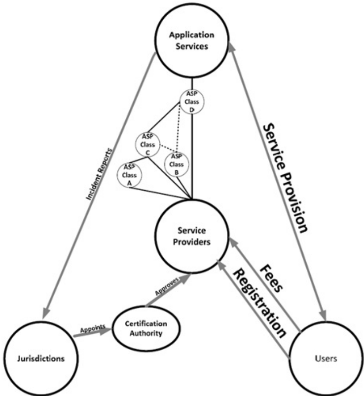
Obrázek 1 – Architektura aplikační služby TARV VPF (Obrázek 2 normy)
