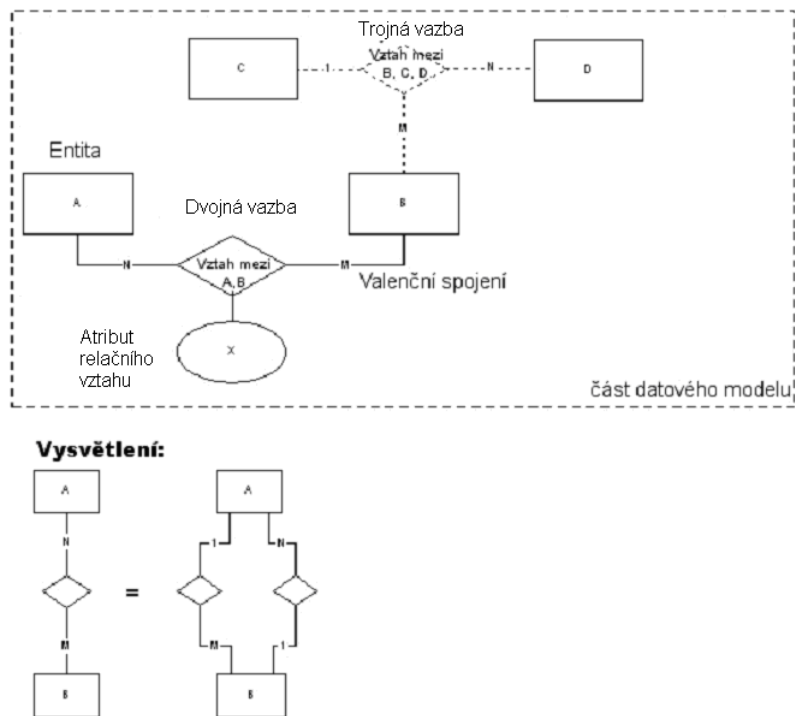
Obrázek 1 - Příklad datového modelu záznam
