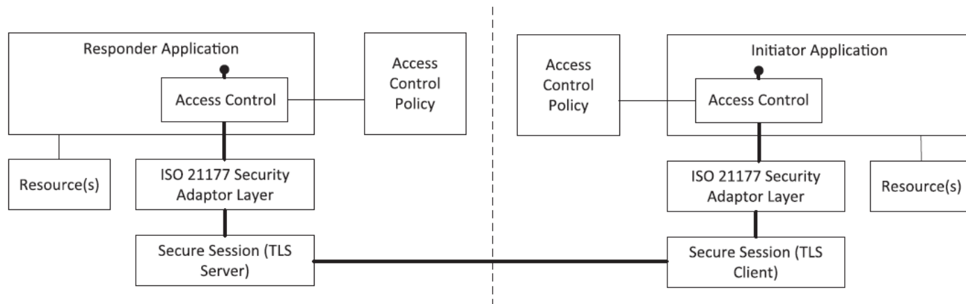
Obrázek 1 (obr. 7 normy): Logická architektura
