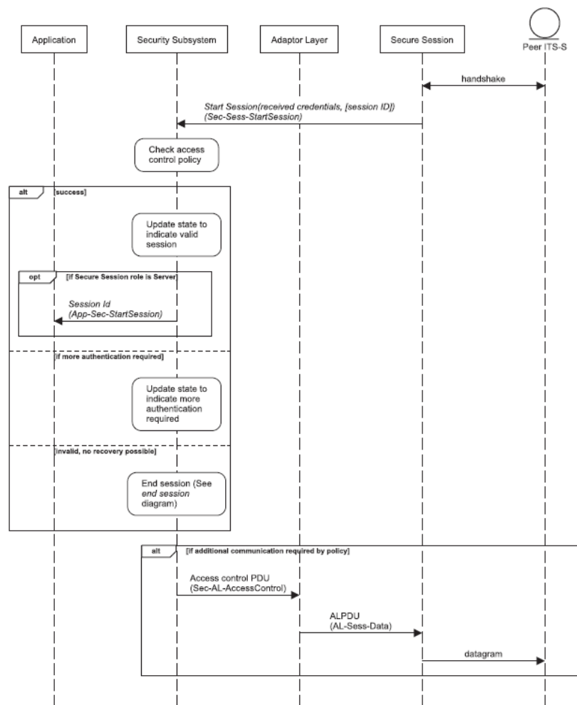
Obrázek 3 (obr. 12 normy): Sekvenční diagram zahájení relace
