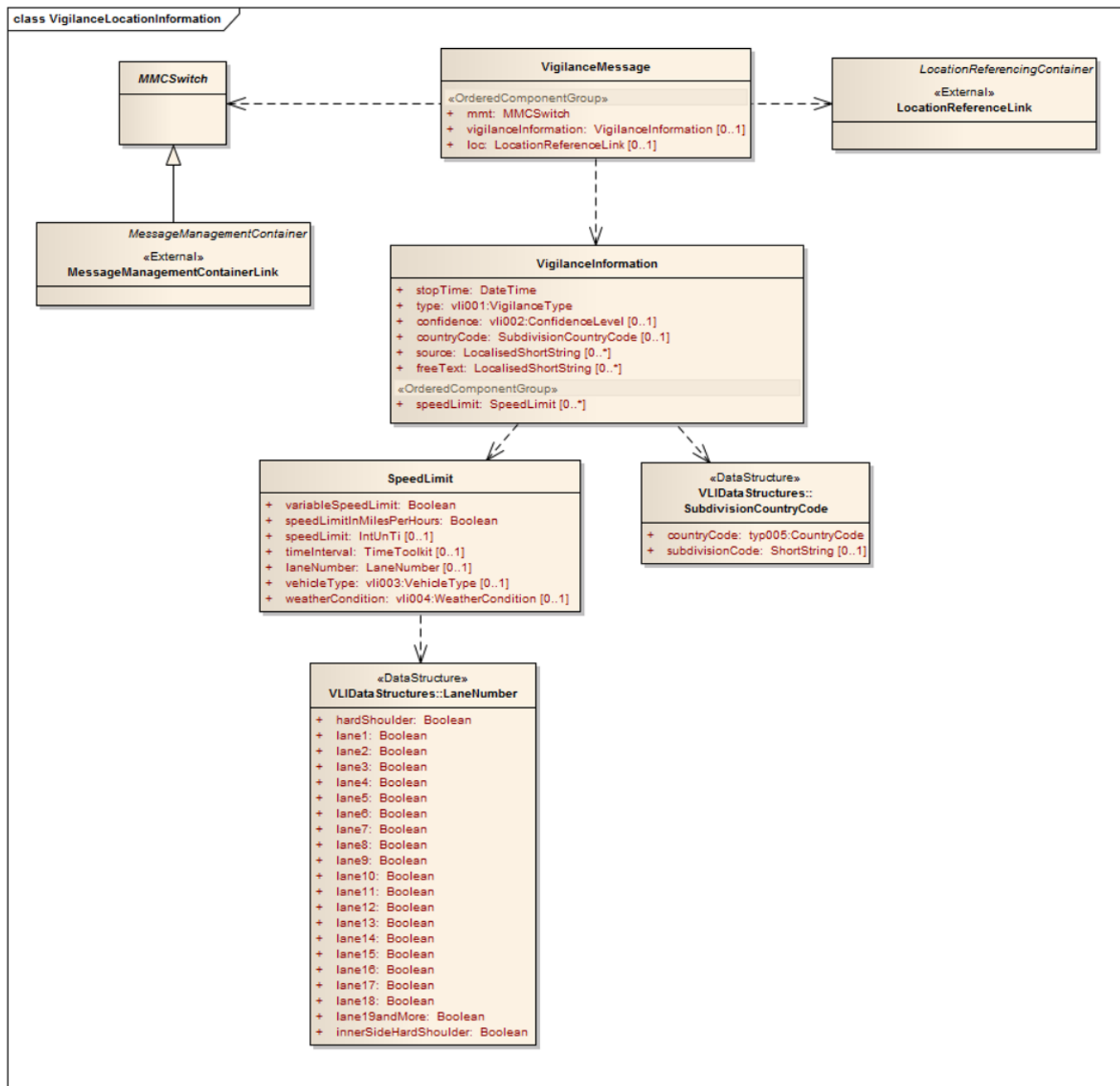
Obrázek 1 - UML model tříd aplikace VLI (obrázek 2 normy)
