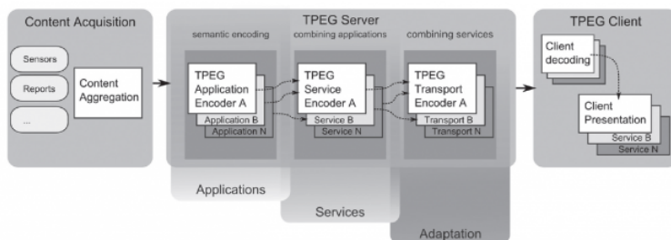
Obrázek 1 - Hierarchie multiplexu TPEG (obrázek 3 dokumentu)
