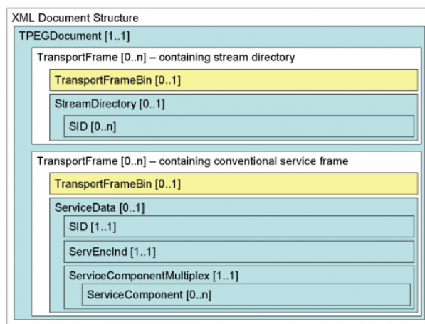
Obrázek 3 - XML Struktura TPEG (obrázek B.1 dokumentu)
