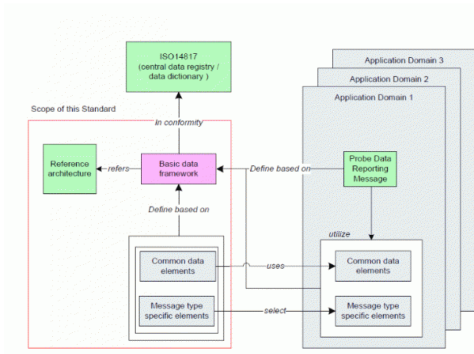
Obrázek 1 – Předmět normy
