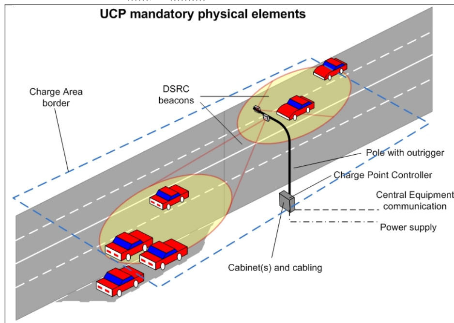
Obrázek 1 - Typické prvky mýtného DSRC bodu m
